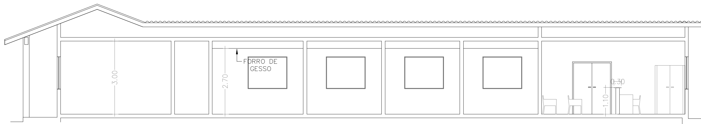
CORTE A-A ESC.: 1:75
