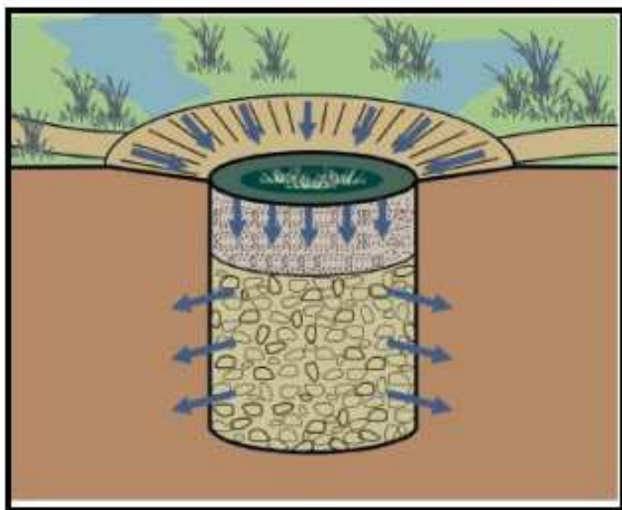
Poço de infiltração
